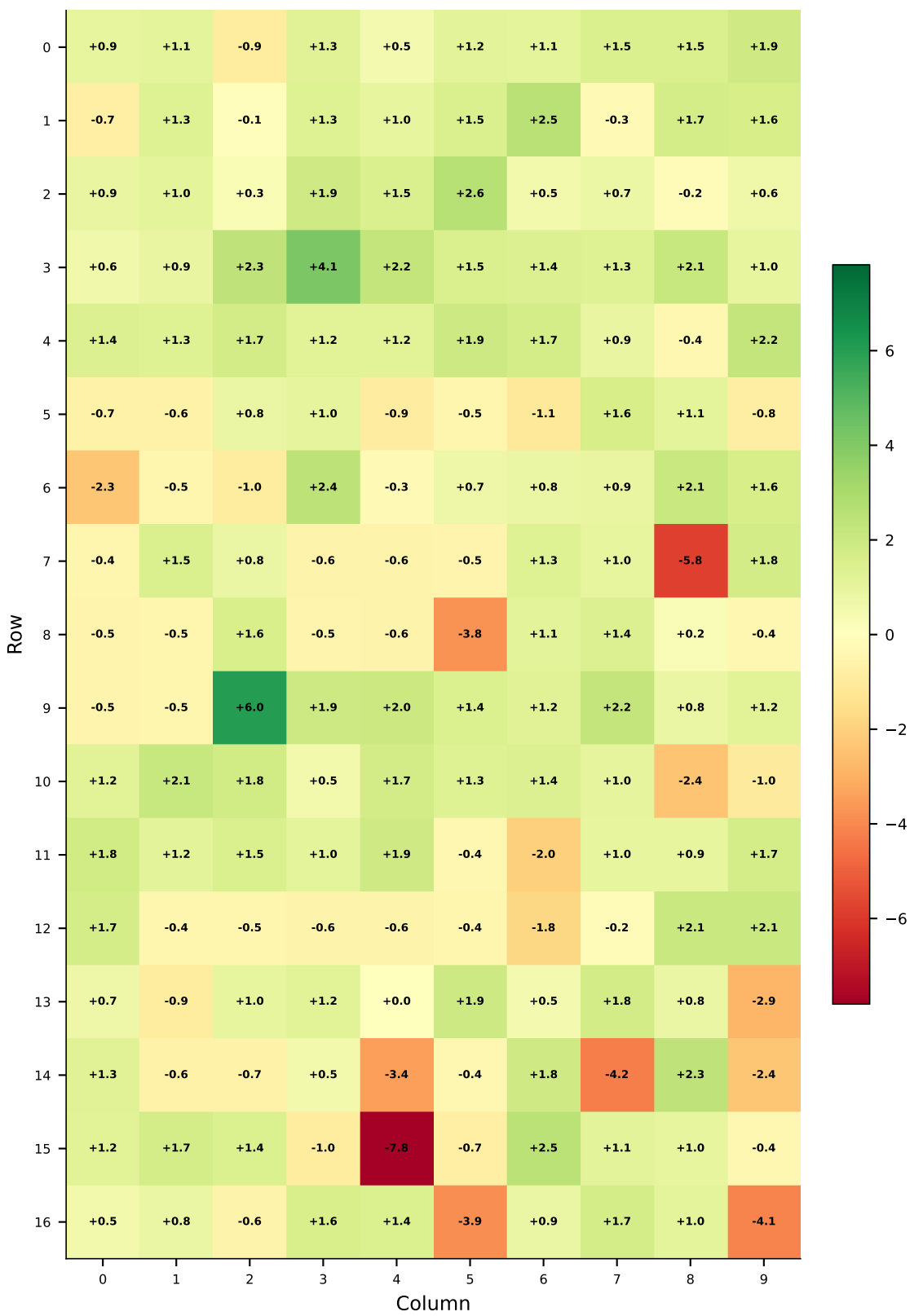
\Delta MAPE (pp)
