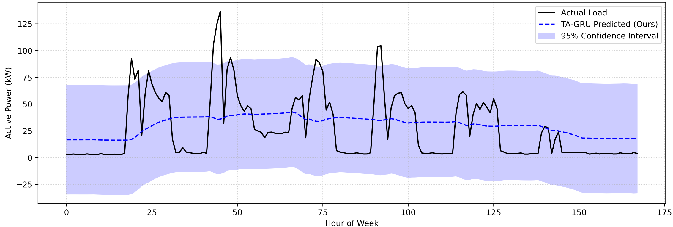
TA-GRU 7-Day Load Forecast vs Actual (UCI Steel Dataset)
