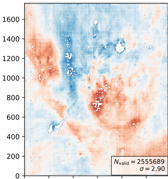
[\text{NII}] \lambda 6583
