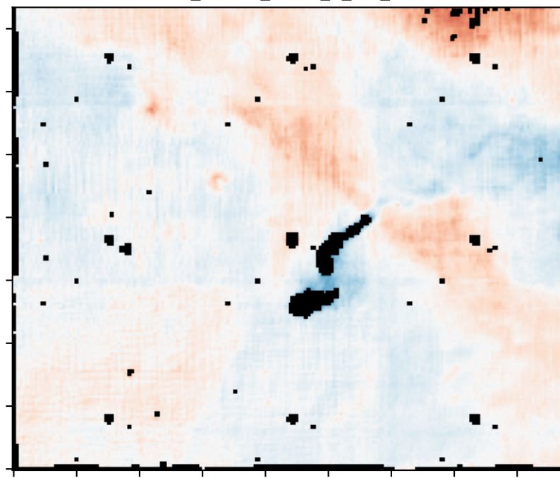
H_I-6563_mask_0_bin_4
