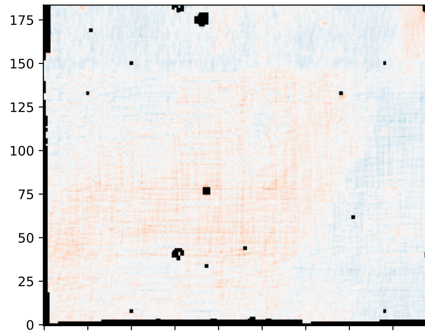
H_I-6563_mask_0_bin_8
