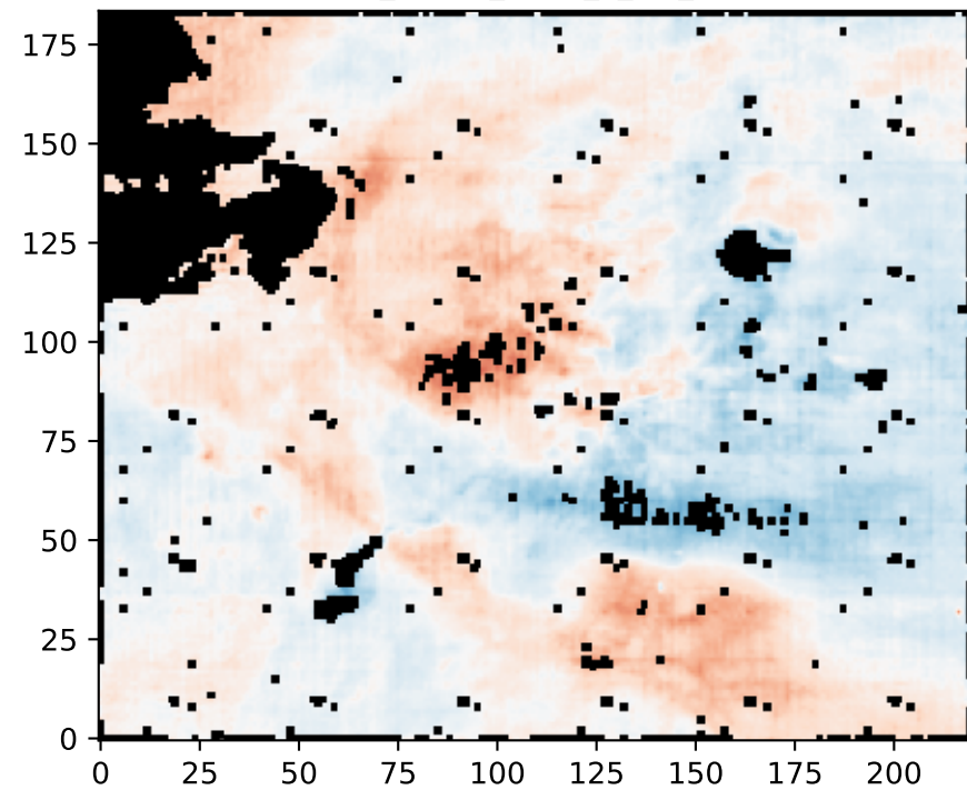
H_I-6563_mask_0_bin_8
