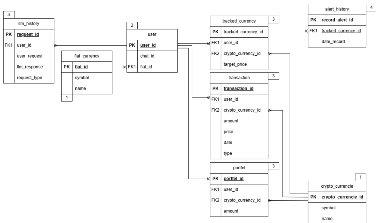
Рисунок 1. Схема базы данных
