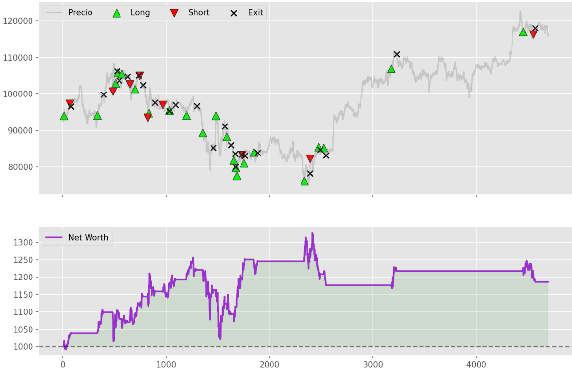
Operativa TEMPORAL-AE (Seed 789) | Retorno: 18.59%
