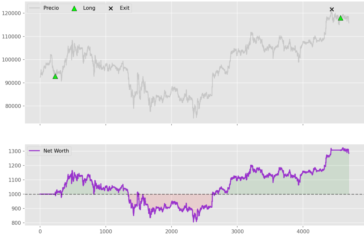
Operativa TRANSFORMER (Seed 456) | Retorno: 28.50%
