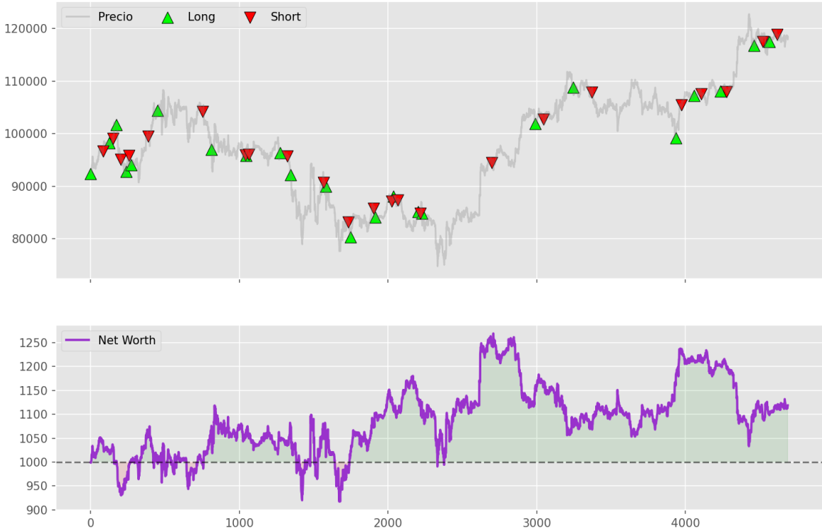
Operativa COMBINADO (Seed 42) | Retorno: 11.90%
