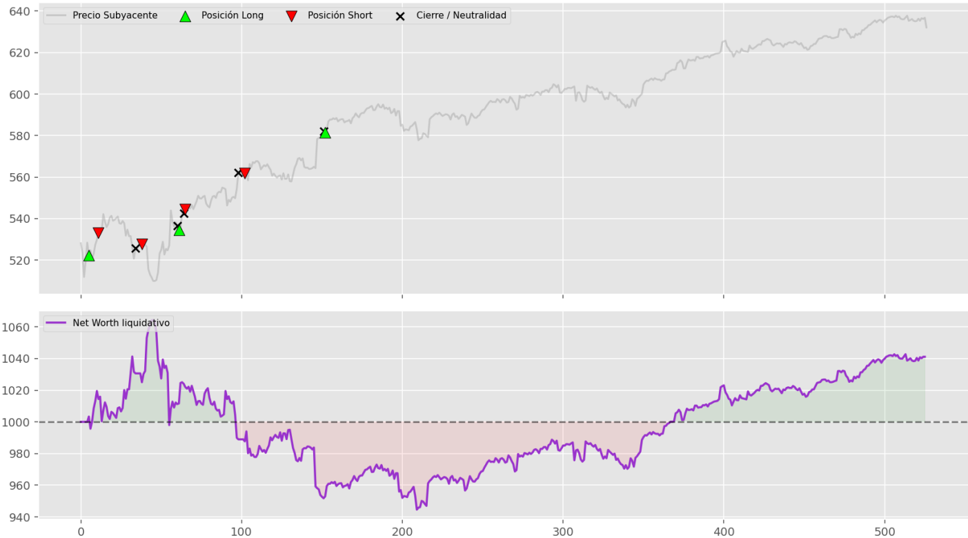
Espacio SRL: CPC | Semilla Estocástica: 123 | Rentabilidad: 4.11%
