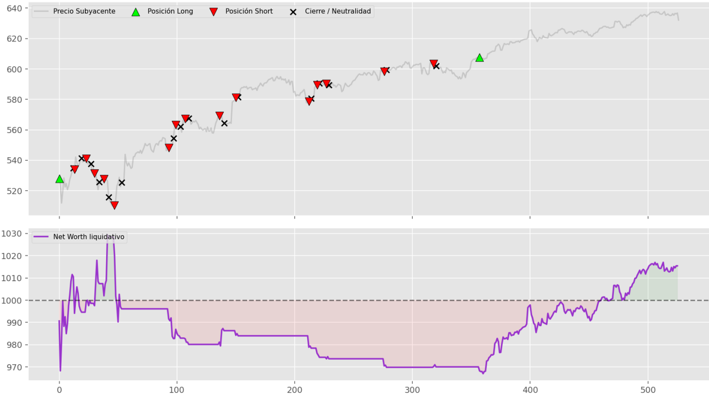
Espacio SRL: CPC | Semilla Estocástica: 42 | Rentabilidad: 1.54%
