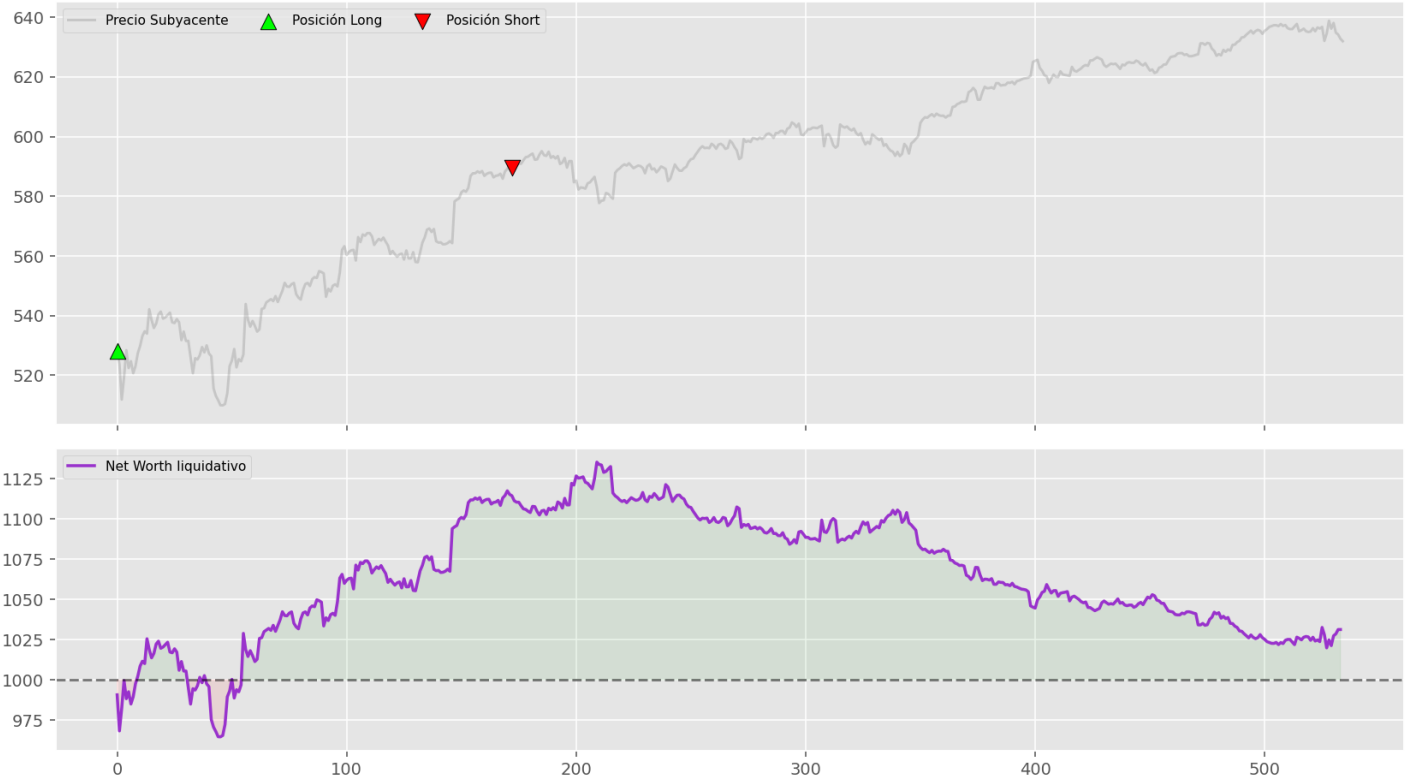
Espacio SRL: TRANSFORMER | Semilla Estocástica: 1011 | Rentabilidad: 3.12%
