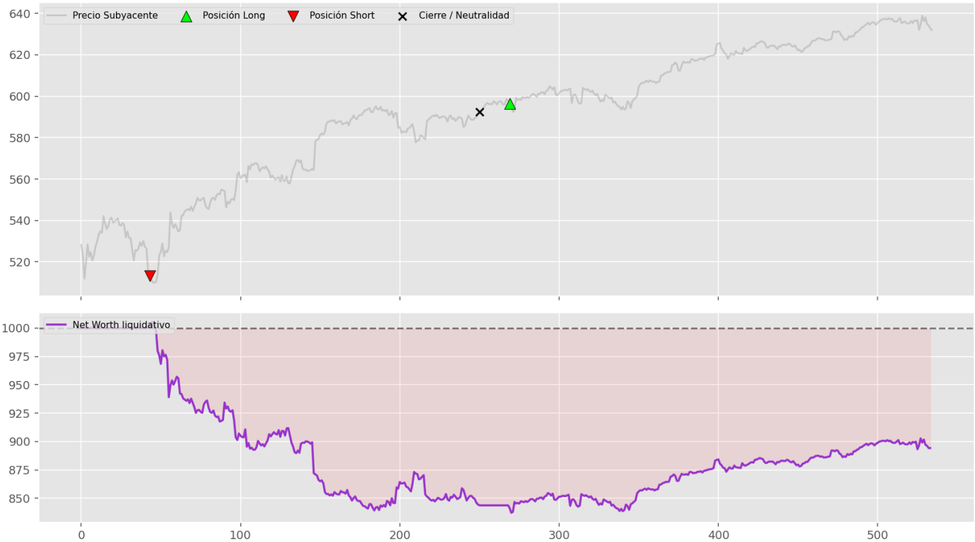
Espacio SRL: TRANSFORMER | Semilla Estocástica: 789 | Rentabilidad: -10.57%
