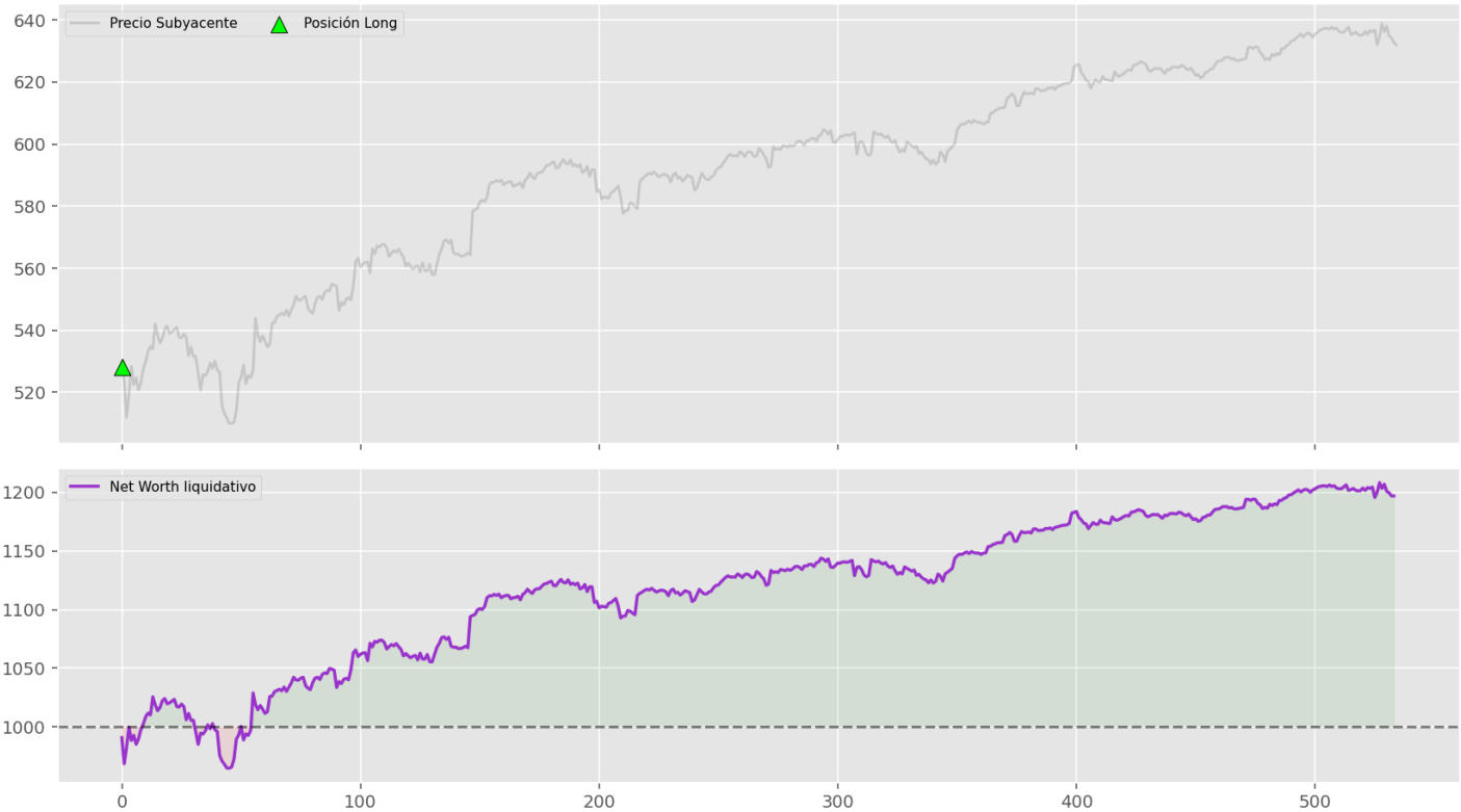
Espacio SRL: TRANSFORMER | Semilla Estocástica: 123 | Rentabilidad: 19.70%
