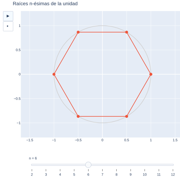
Figura 9: Raíces n -ésimas de la unidad con un deslizador en n : al variar n cambia el número de vértices del polígono regular inscrito en la circunferencia unidad. [ver versión interactiva]
