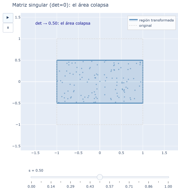
Figura 12: Cuando \det A \rightarrow 0 la transformación aplasta el área a cero: una matriz singular colapsa el espacio a una dimensión menor. [ver versión interactiva]
