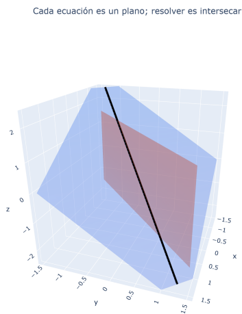
Figura 5: Cada ecuación de un sistema es un plano en \mathbb{R}^3 ; la solución es su intersección (aquí, una recta).
