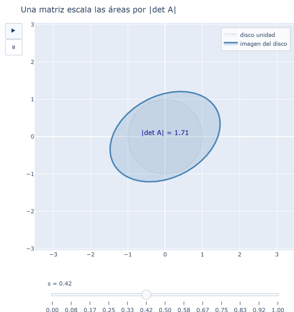
Figura 8: Una matriz 2 \times 2 transforma el disco unidad en una elipse, multiplicando el área por |\det A| .
