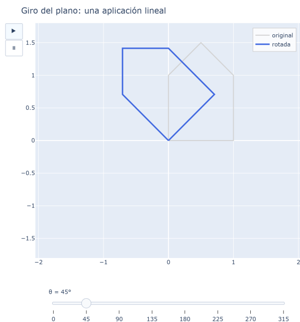
Figura 7: El giro del plano es una aplicación lineal: cada vector se transforma girándolo el mismo ángulo (aquí, una figura y su rotada). [ver versión interactiva]
