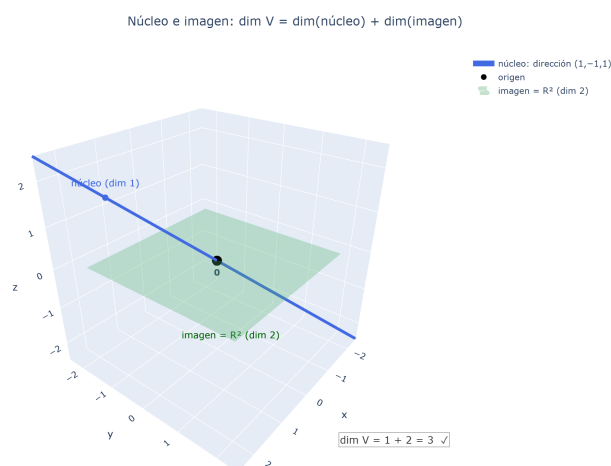
Figura 9: Núcleo e imagen de una aplicación lineal: lo que se colapsa (el núcleo, aquí una recta) y lo que se conserva; \dim V = \dim(\text{núcleo}) + \dim(\text{imagen}) .
