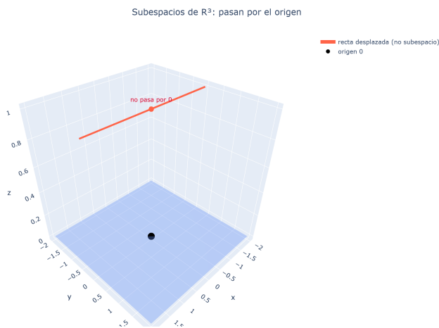
Figura 4: Un subespacio de \mathbb{R}^3 pasa por el origen (un plano, aquí); una recta desplazada que no pasa por 0 no es subespacio.
