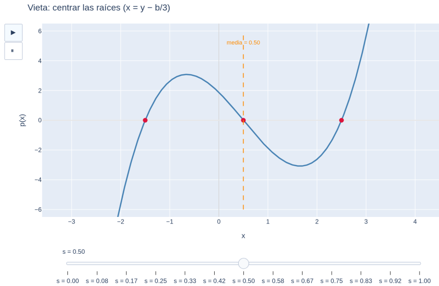
Figura 8: La sustitución x = y - b/3 centra las raíces en su media (elimina el término cuadrático) — el primer paso del método de Cardano. [ver versión interactiva]
