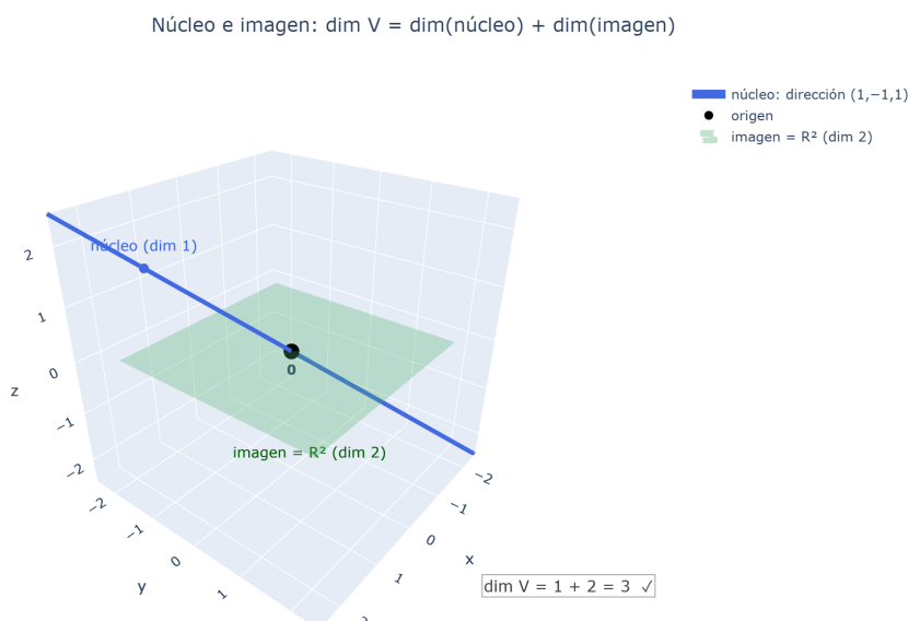
Figura 9: Núcleo e imagen de una aplicación lineal: lo que se colapsa (el núcleo, aquí una recta) y lo que se conserva; \dim V = \dim(\text{núcleo}) + \dim(\text{imagen}) .
