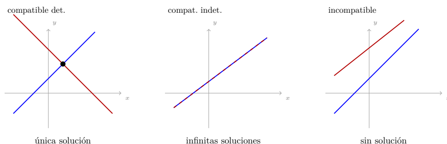
Figura 2: Los tres casos de un sistema 2 \times 2 , geoméricamente: rectas que se cortan (única solución), coincidentes (infinitas) o paralelas (sin solución).
