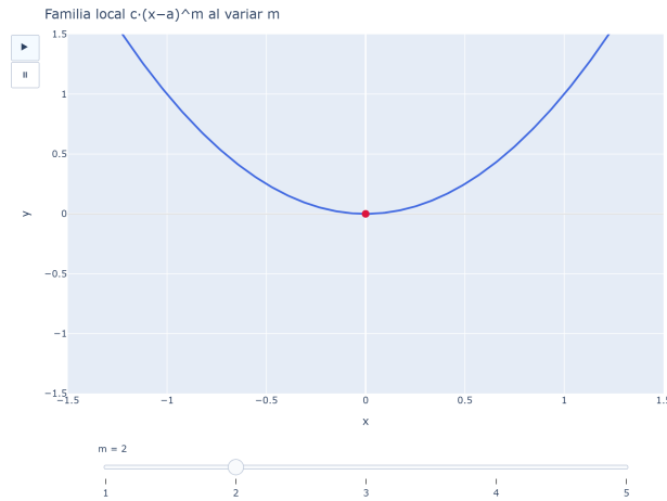
Figura 2: Familia local c(x-a)^m al variar m = 1, 2, 3, \dots : el tránsito cruce ( m impar) rebote ( m par) y el aplanamiento creciente del contacto. [ver versión interactiva]
