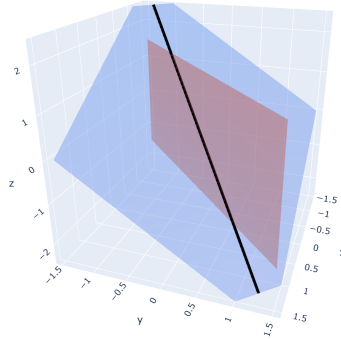
Figura 5: Cada ecuación de un sistema es un plano en \mathbb{R}^3 ; la solución es su intersección (aquí, una recta).
