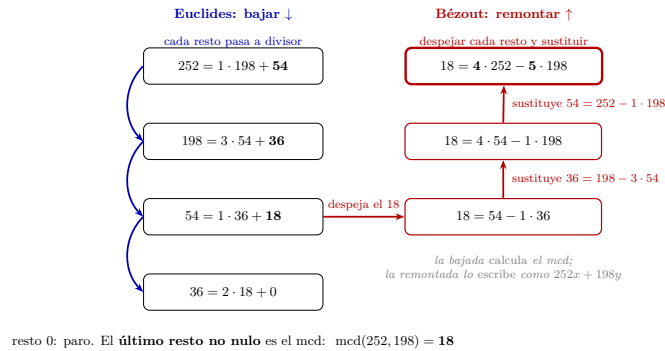
Figura 2: La imagen mental del algoritmo extendido, con el Ejemplo 1.8: Euclides baja (cada resto pasa a divisor, hasta el último resto no nulo — el mcd) y Bézout remonta (despeja el mcd de la penúltima división y sustituye los restos hacia arriba, hasta escribirlo como combinación de los datos originales).
