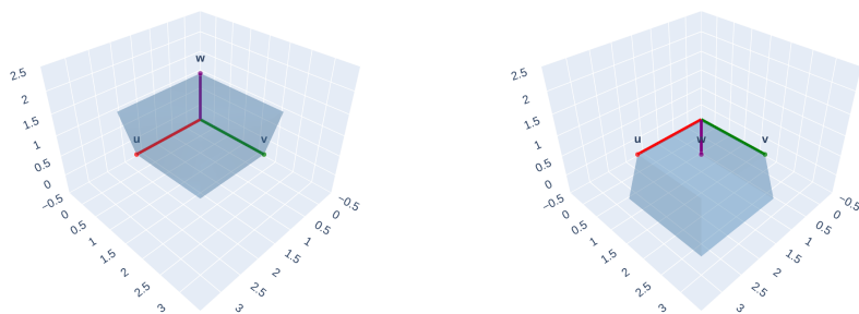
Figura 23: Coplanariedad \iff volumen 0: cuando el tercer vector se acerca al plano de los otros dos, el paralelepípedo se aplasta y ||[u, v, w]|| \rightarrow 0 .
