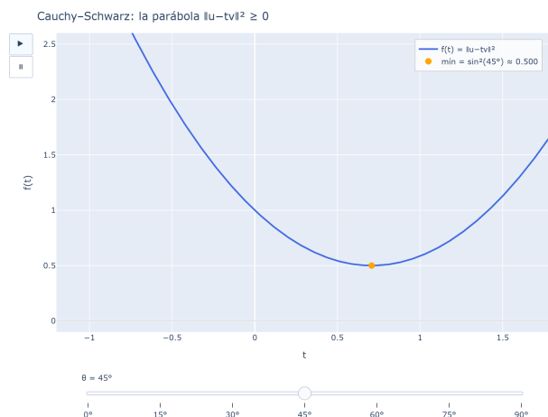
Figura 9: Cauchy–Schwarz, visto: f(t) = \|u - tv\|^2 es una parábola que nunca baja del eje; que su discriminante sea \leq 0 es la desigualdad, y toca el eje (igualdad) solo si u, v son proporcionales.
