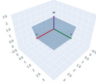
Figura 20: Coplanariedad \iff volumen 0: cuando el tercer vector se acerca al plano de los otros dos, el paralelepípedo se aplasta y |[u, v, w]| \rightarrow 0 . [ver versión interactiva]
