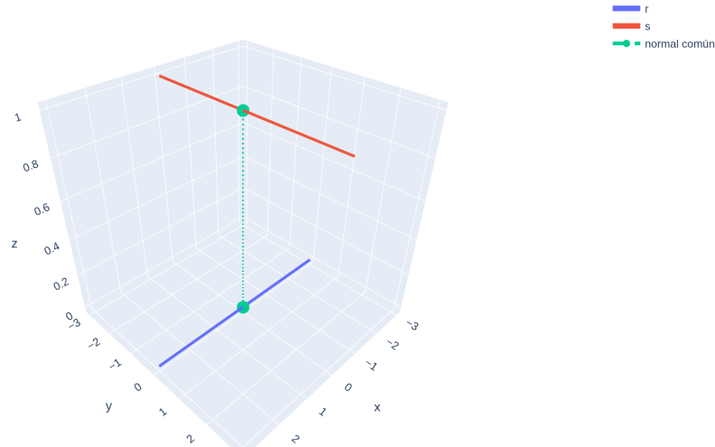
Figura 22: Dos rectas cruzadas r, s y el segmento de la normal común que realiza la distancia mínima; al girar la vista se ve que no se cortan.
