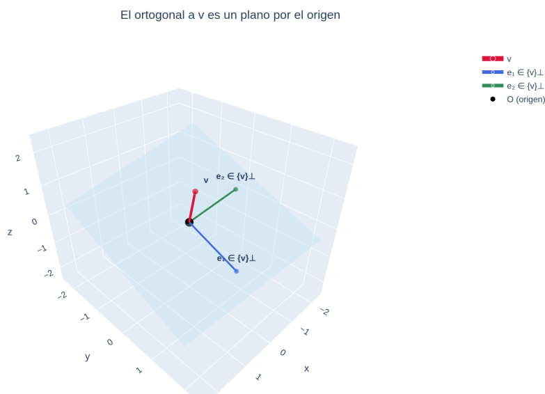
Figura 13: El ortogonal a un vector no nulo v es un plano por el origen: \{v\}^\perp = \{u : u \cdot v = 0\} . Es la base de la idea de “normal” de un plano.
