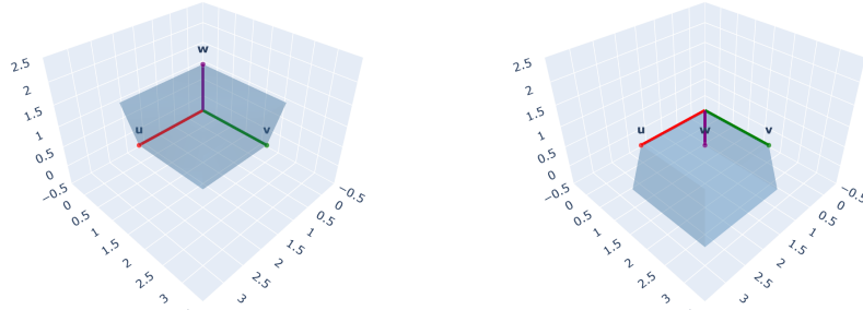
Figura 19: Coplanariedad \iff volumen 0: cuando el tercer vector se acerca al plano de los otros dos, el paralelepípedo se aplasta y |[u,v,w]| \rightarrow 0 .
