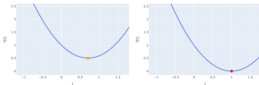
Figura 9: Cauchy–Schwarz, visto: f(t) = \|u - tv\|^2 es una parábola que nunca baja del eje; que su discriminante sea \leq 0 es la desigualdad, y toca el eje (igualdad) solo si u, v son proporcionales.
