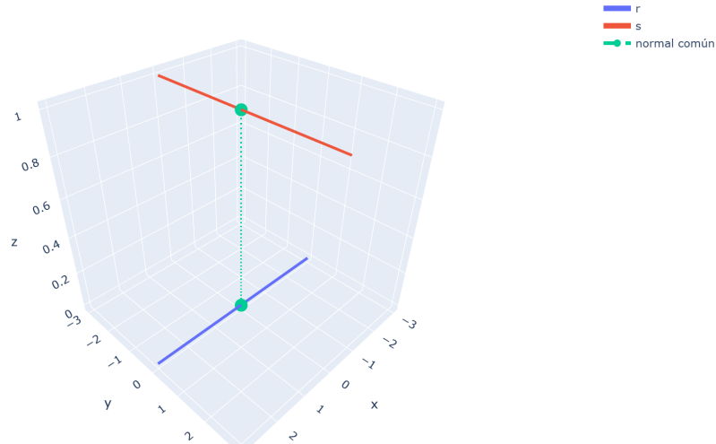
Figura 21: Dos rectas cruzadas r, s y el segmento de la normal común que realiza la distancia mínima; al girar la vista se ve que no se cortan.
