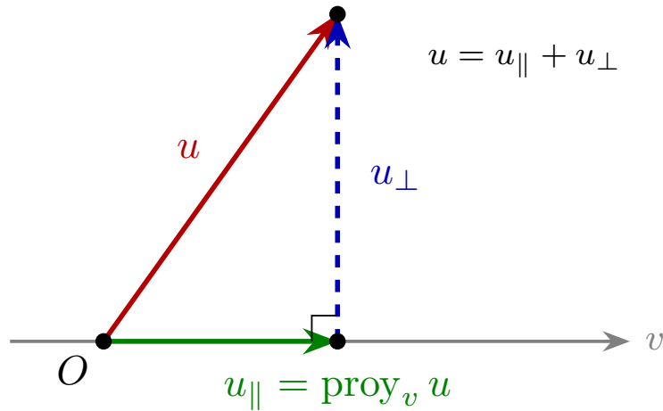
Figura 13: Descomposición ortogonal: u = u_{\parallel} + u_{\perp} , con u_{\parallel} = \text{proy}_v u la componente sobre v y u_{\perp} la perpendicular.
