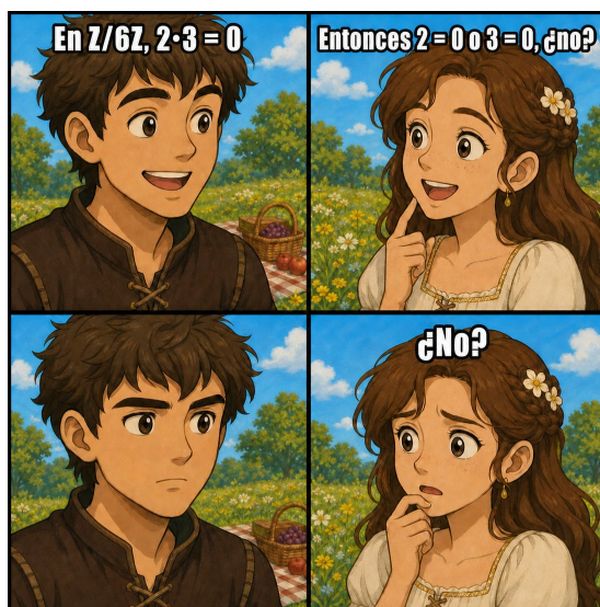
Figura 4: El reflejo que esta sección desmonta: en \mathbb{Z} (¡o en \mathbb{R} !) un producto nulo delata un factor nulo, pero en \mathbb{Z}/6\mathbb{Z} es 2 \cdot 3 = \bar{0} con ambos factores no nulos — divisores de cero, exactamente lo que el Teorema 3.10 detecta con \text{mcd} > 1 .
