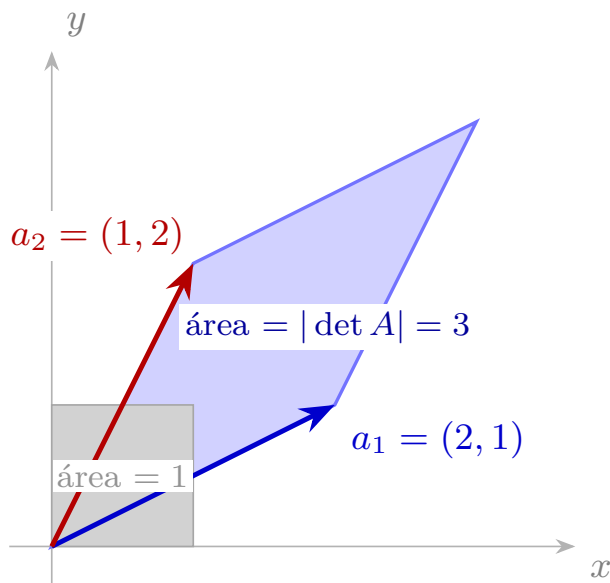
Figura 10: El determinante como factor de área: la matriz A lleva el cuadrado unidad (área 1) a un paralelogramo de área |\det A| .
