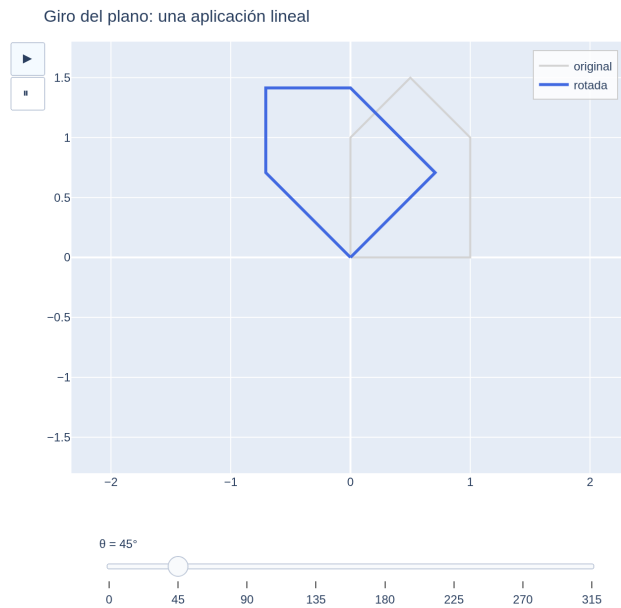
Figura 7: El giro del plano es una aplicación lineal: cada vector se transforma girándolo el mismo ángulo (aquí, una figura y su rotada). [ver versión interactiva]
