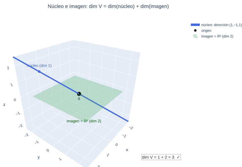
Figura 9: Núcleo e imagen de una aplicación lineal: lo que se colapsa (el núcleo, aquí una recta) y lo que se conserva; \dim V = \dim(\text{núcleo}) + \dim(\text{imagen}) .
