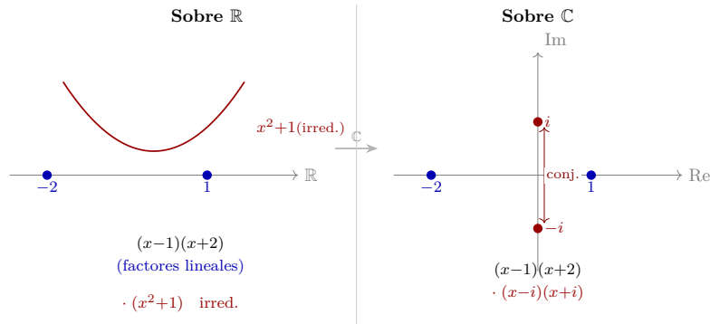
Figura 6: Sobre \mathbb{R} un polinomio se factoriza en lineales y cuadráticos irreducibles; sobre \mathbb{C} esos cuadráticos se abren en pares de raíces conjugadas.
