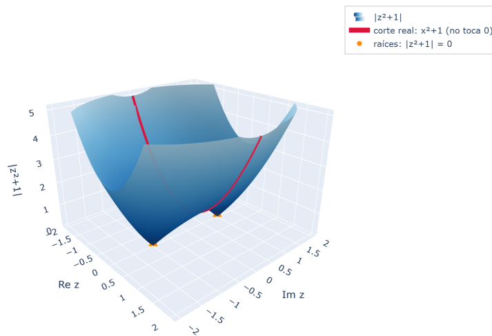
Figura 5: La dimensión extra: el paisaje |z^2 + 1| sobre el plano complejo. El corte sobre el eje real (rojo) es la parábola x^2 + 1 , que no toca el suelo; el paisaje completo sí lo toca, exactamente en las raíces \pm i (naranja).
