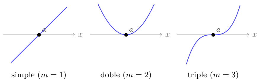
Figura 1: Tres comportamientos en el corte x = a según la multiplicidad m : simple ( m = 1 ) cruza con pendiente no nula; doble ( m = 2 ) toca y rebota sin cambiar de signo; triple ( m = 3 ) cruza aplanándose. Regla: m impar cruza, m par rebota.
