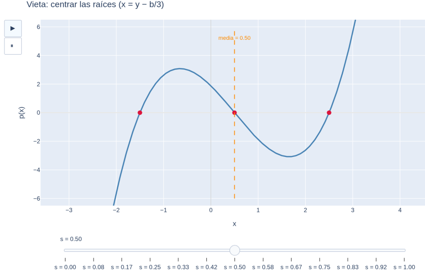
Figura 7: La sustitución x = y - b/3 centra las raíces en su media (elimina el término cuadrático) — el primer paso del método de Cardano.
