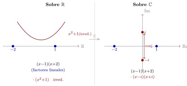
Figura 6: Sobre \mathbb{R} un polinomio se factoriza en lineales y cuadráticos irreducibles; sobre \mathbb{C} esos cuadráticos se abren en pares de raíces conjugadas.
