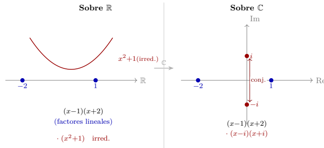
Figura 5: Sobre \mathbb{R} un polinomio se factoriza en lineales y cuadráticos irreducibles; sobre \mathbb{C} esos cuadráticos se abren en pares de raíces conjugadas.
