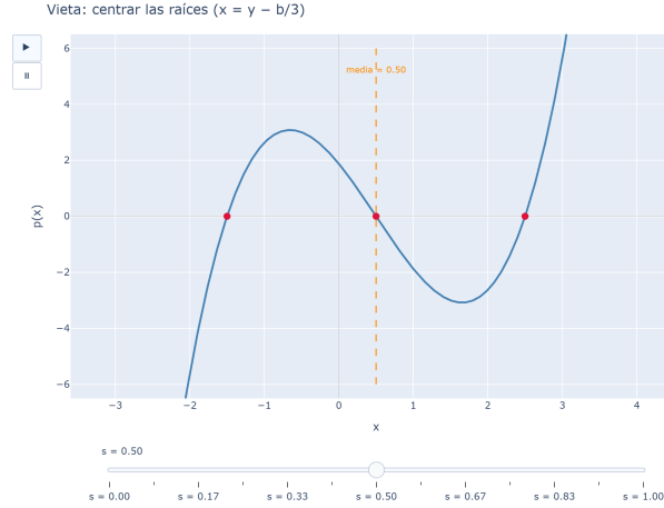
Figura 6: La sustitución x = y - b/3 centra las raíces en su media (elimina el término cuadrático) — el primer paso del método de Cardano. [ver versión interactiva]
