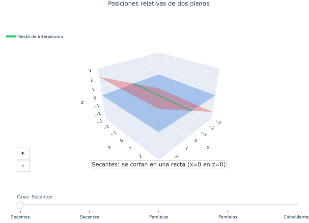
Figura 7: Posiciones relativas de dos planos en el espacio: se cortan en una recta (secantes), son paralelos o coinciden — con un deslizador que recorre los casos. [ver versión interactiva]
