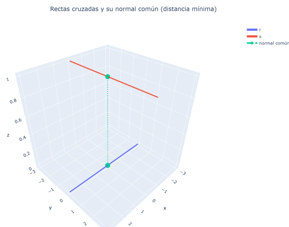
Figura 21: Dos rectas cruzadas r, s y el segmento de la normal común que realiza la distancia mínima; al girar la vista se ve que no se cortan. [ver versión interactiva]
