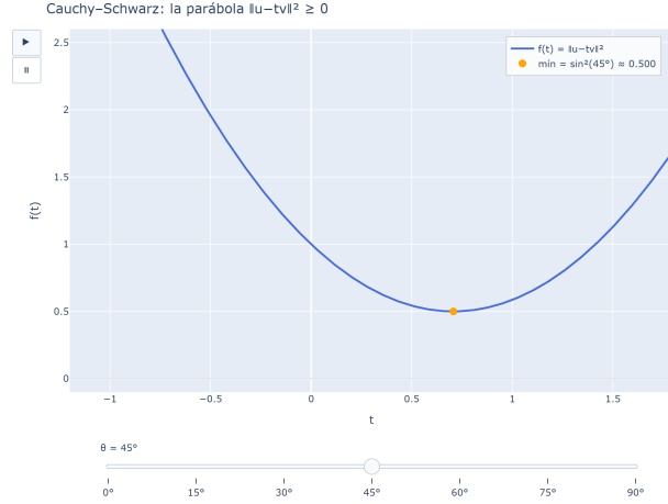
Figura 9: Cauchy–Schwarz, visto: f(t) = \|u - tv\|^2 es una parábola que nunca baja del eje; que su discriminante sea \leq 0 es la desigualdad, y toca el eje (igualdad) solo si u, v son proporcionales.
