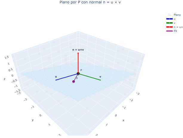
Figura 20: Plano por P con directores u, v y la normal n = u \times v saliendo del plano; un punto genérico X con PX contenido en el plano (perpendicular a n ). [ver versión interactiva]
