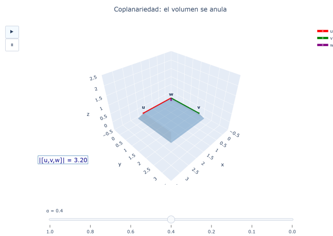
Figura 19: Coplanariedad \iff volumen 0: cuando el tercer vector se acerca al plano de los otros dos, el paralelepípedo se aplasta y |[u, v, w]| \rightarrow 0 . [ver versión interactiva]
