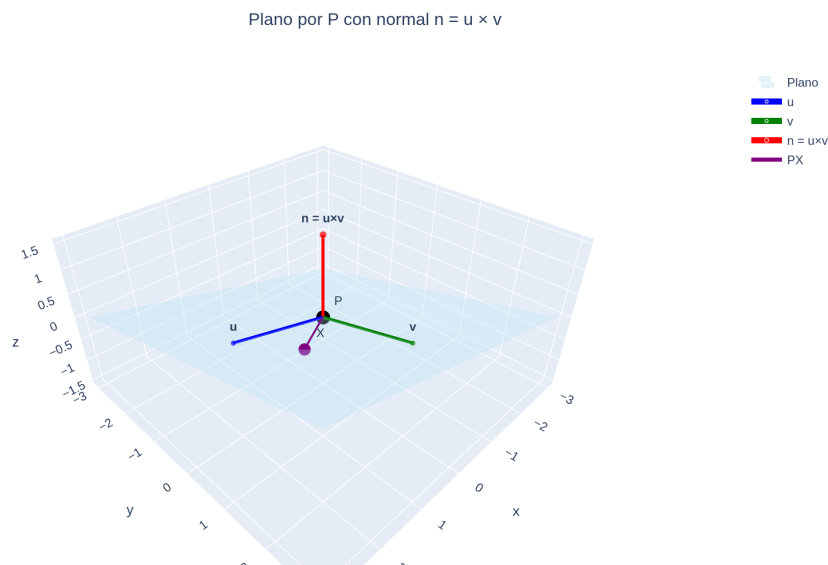
Figura 21: Plano por P con directores u, v y la normal n = u \times v saliendo del plano; un punto genérico X con \vec{PX} contenido en el plano (perpendicular a n ).
