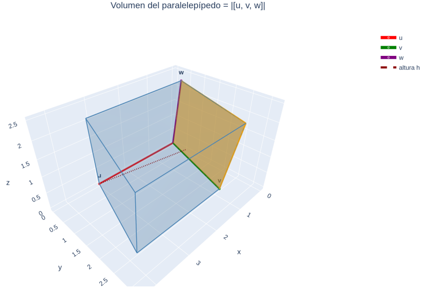
Figura 19: Paralelepípedo de aristas u, v, w desde un vértice común: base el paralelogramo de v, w (área ||v \times w|| ) y altura ||\text{proy}_n u|| con n = v \times w ; coplanario, se aplasta a un plano (volumen 0).
