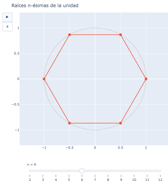
Figura 9: Raíces n -ésimas de la unidad con un deslizador en n : al variar n cambia el número de vértices del polígono regular inscrito en la circunferencia unidad. [ver versión interactiva]
