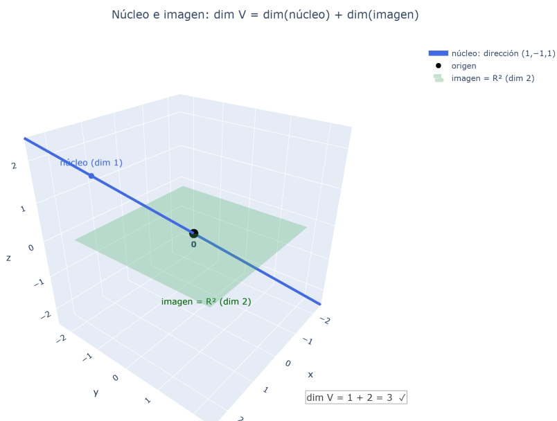
Figura 9: Núcleo e imagen de una aplicación lineal: lo que se colapsa (el núcleo, aquí una recta) y lo que se conserva; \dim V = \dim(\text{núcleo}) + \dim(\text{imagen}) .
