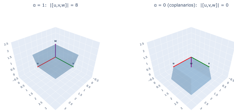
Figura 19: Coplanariedad \iff volumen 0: cuando el tercer vector se acerca al plano de los otros dos, el paralelepípedo se aplasta y |[u, v, w]| \rightarrow 0 . [ver versión interactiva]
