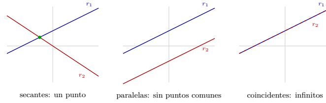
Figura 6: Posiciones relativas de dos rectas en el plano (versión interactiva: arrastra los puntos de r_2 ): se cortan en un punto (secantes), no se cortan (paralelas) o coinciden.
