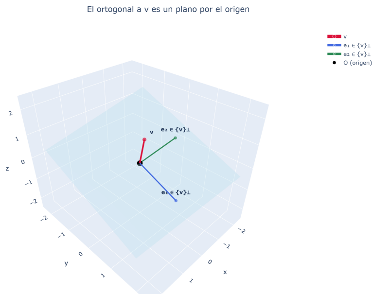
Figura 12: El ortogonal a un vector no nulo v es un plano por el origen: \{v\}^\perp = \{u : u \cdot v = 0\} . Es la base de la idea de “normal” de un plano.
