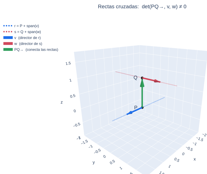
Figura 9: Las tres columnas del determinante de la Proposición 5.2.5, sobre el par cruzado del Ejemplo 5.2.6: los directores v y w saliendo de P y de Q , y el vector \vec{PQ} que conecta las dos rectas. Que los tres no sean coplanarios es que el determinante no se anule; girando la figura se ve que r y s no se cortan, aunque de frente lo parezca.
