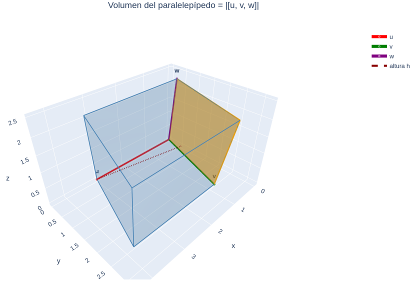
Figura 20: Paralelepípedo de aristas u, v, w desde un vértice común: base el paralelogramo de v, w (área ||v \times w|| ) y altura ||\text{proy}_n u|| con n = v \times w ; coplanario, se aplasta a un plano (volumen 0).
