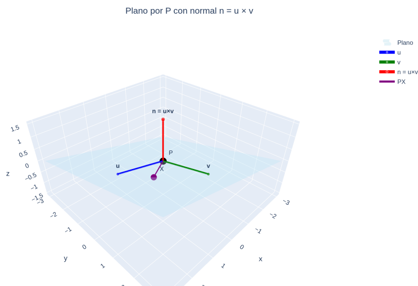
Figura 22: Plano por P con directores u, v y la normal n = u \times v saliendo del plano; un punto genérico X con \vec{PX} contenido en el plano (perpendicular a n ).
