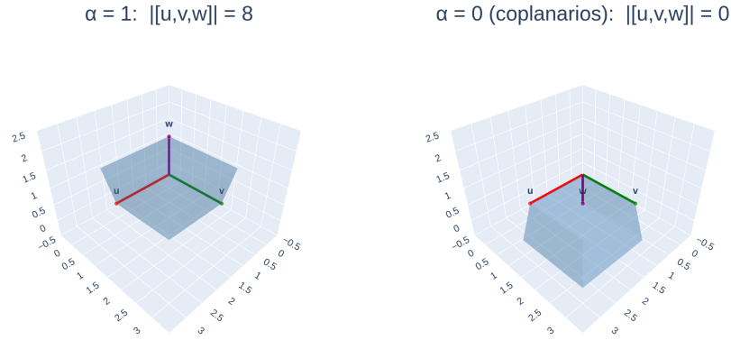
Figura 21: Coplanariedad \iff volumen 0: cuando el tercer vector se acerca al plano de los otros dos, el paralelepípedo se aplasta y ||[u, v, w]|| \rightarrow 0 .
