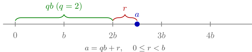
Figura 1: La división euclídea en la recta: a cae entre dos múltiplos consecutivos de b ; el cociente q los cuenta y el resto r es lo que sobra ( 0 \leq r < b ).
