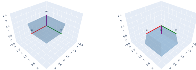
Figura 20: Coplanariedad \iff volumen 0: cuando el tercer vector se acerca al plano de los otros dos, el paralelepípedo se aplasta y |[u, v, w]| \rightarrow 0 .
