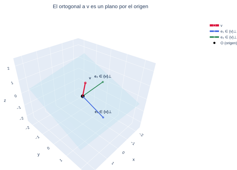
Figura 13: El ortogonal a un vector no nulo v es un plano por el origen: \{v\}^\perp = \{u : u \cdot v = 0\} . Es la base de la idea de “normal” de un plano.
