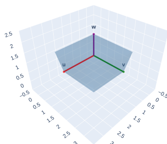
Figura 19: Coplanariedad \iff volumen 0: cuando el tercer vector se acerca al plano de los otros dos, el paralelepípedo se aplasta y |[u, v, w]| \rightarrow 0 .
