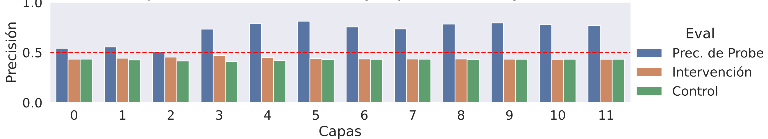
Representaciones Abstractas de Igual y Diferente: Imagenet
