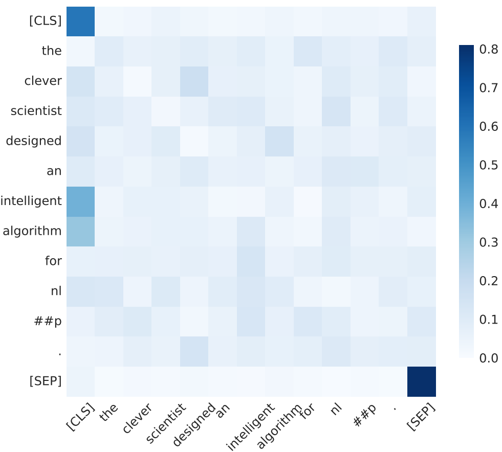
L7-H2: Atención a tokens delimitadores ([CLS]/[SEP])
