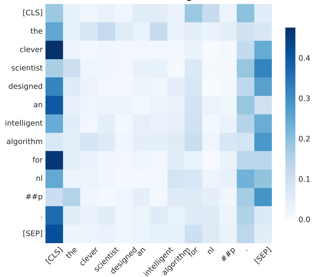
L10-H4: Atención semántica distribuida profunda
