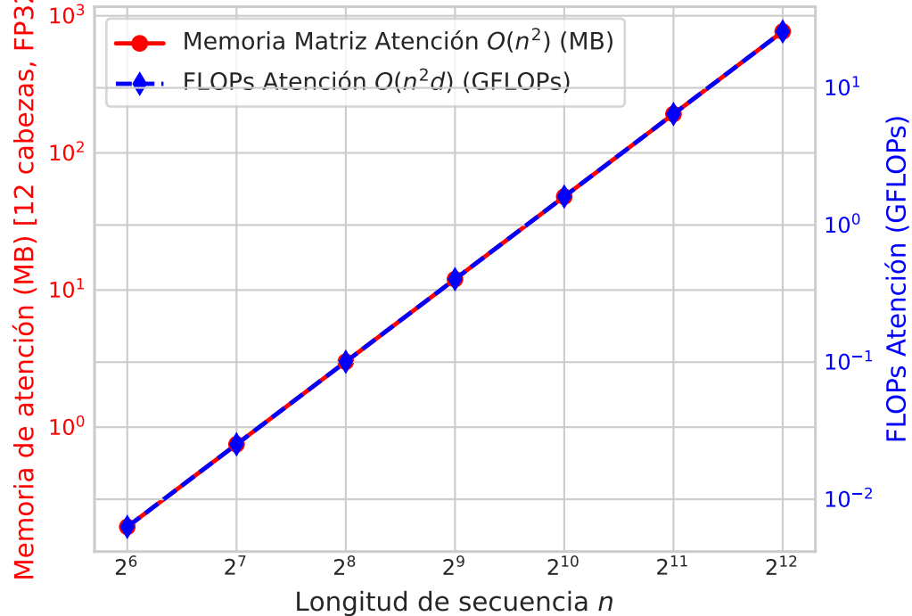
Escalamiento Cuadrático O(n^2) vs Longitud n
