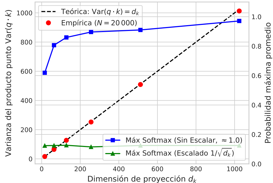
Verificación de Varianza de Scaled Dot-Product
