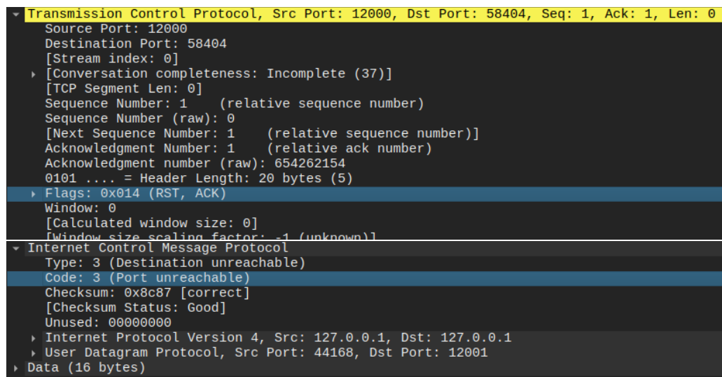
Figura 16: Campos que justifican el rechazo: flags RST y ACK del segmento TCP (arriba) y tipo 3/código 3 del mensaje ICMP (abajo).
