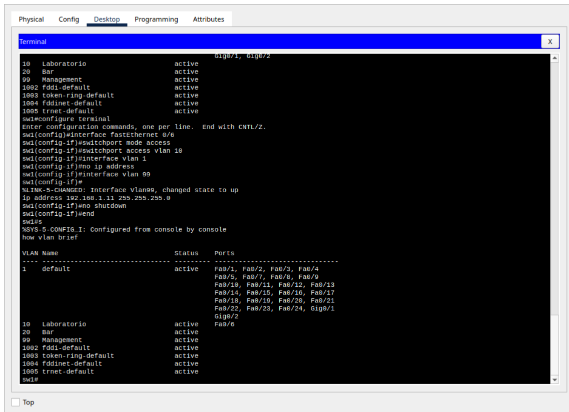
Figura 10: Inciso 1): show vlan brief de sw1, con Fa0/6 asignado a Laboratorio.
