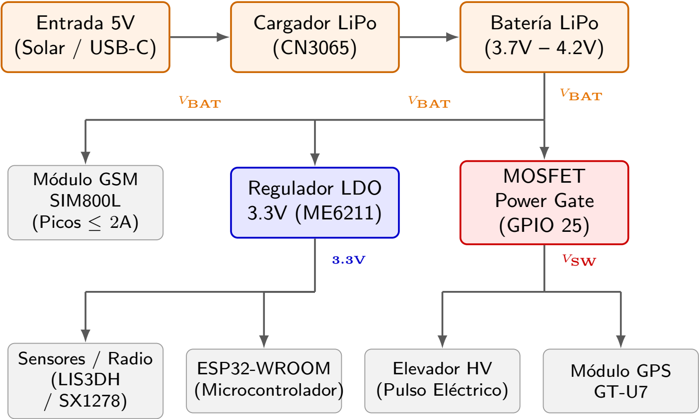
Figura 2: Árbol de distribución de potencia y gestión energética para el sistema DR-VF-01.
