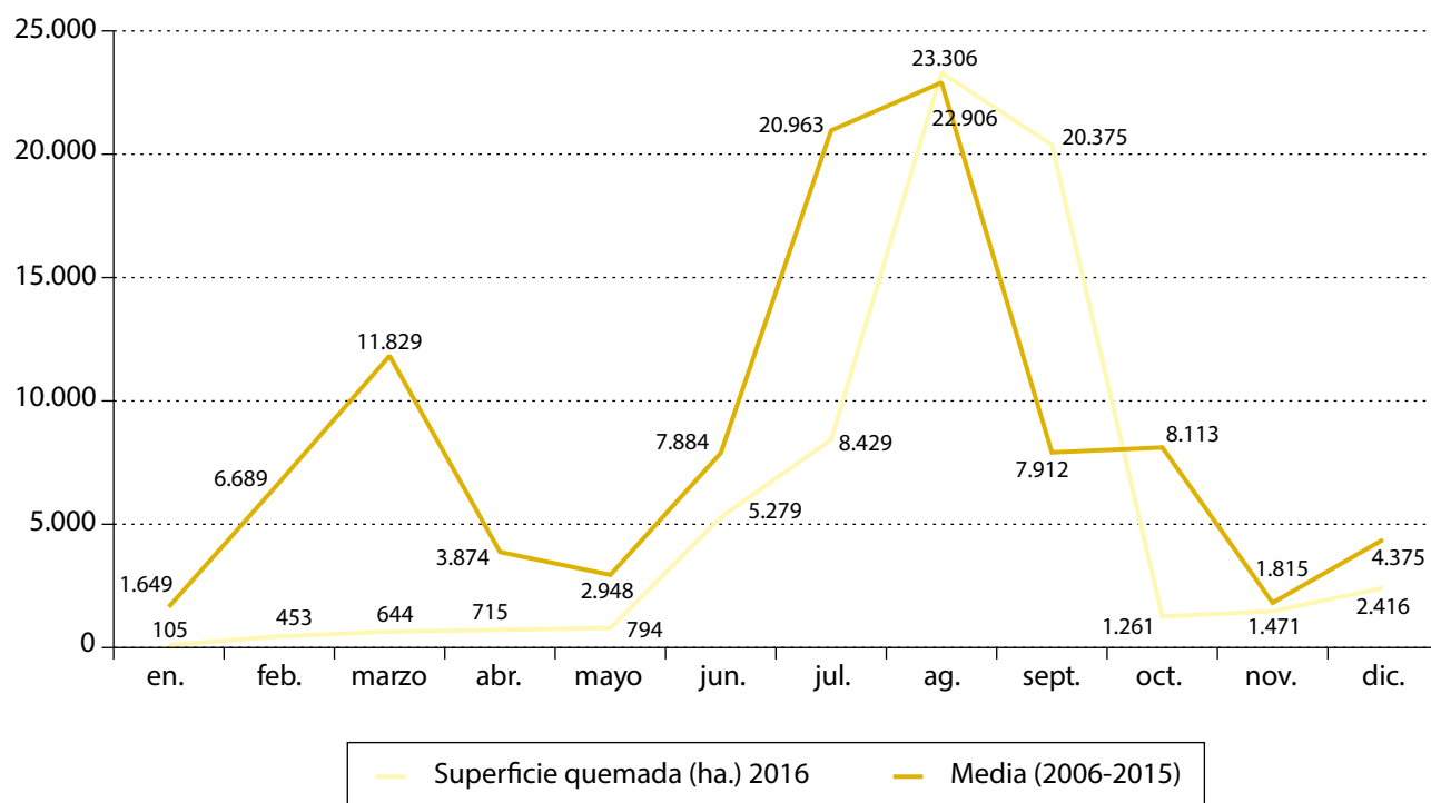
GRÁFICO 6-14. DISTRIBUCIÓN MENSUAL DE SUPERFICIE QUEMADA EN 2016
