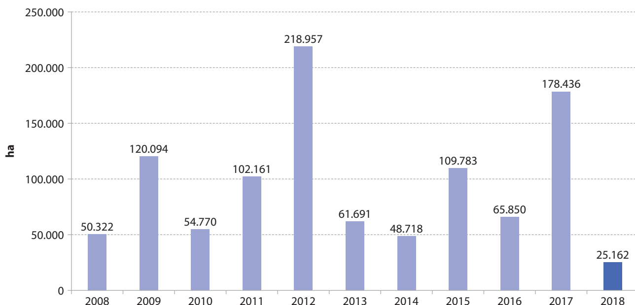
GRÁFICO 6-6-3. SUPERFICIE FORESTAL ANUAL QUEMADA 2008-2018
