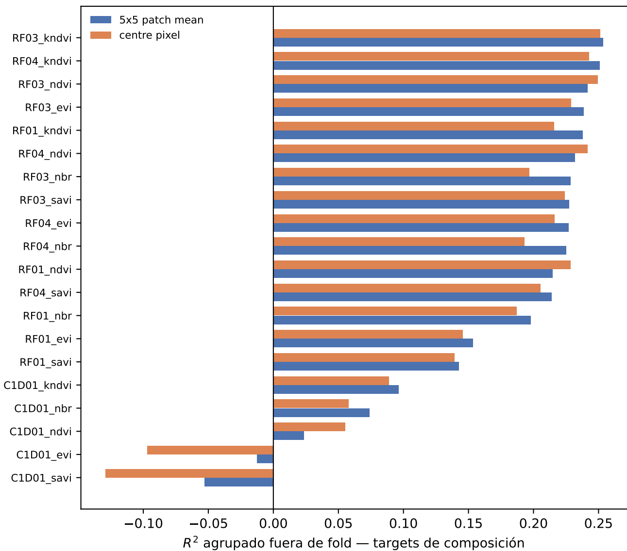
Píxel central contra media 5×5, mismo diseño en todo lo demás
