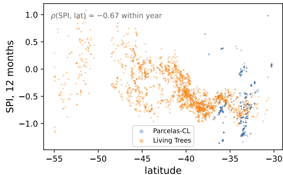
B. SPI tracks latitude
