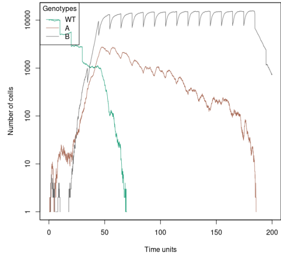
Figura 5.6: Evolución poblacional. Ejemplo 1 terapia adaptativa
