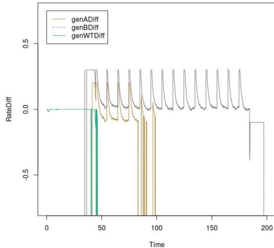
Figura 5.5: Diferencia tasas de nacimiento y muerte. Ejemplo 1 terapia adaptativa
