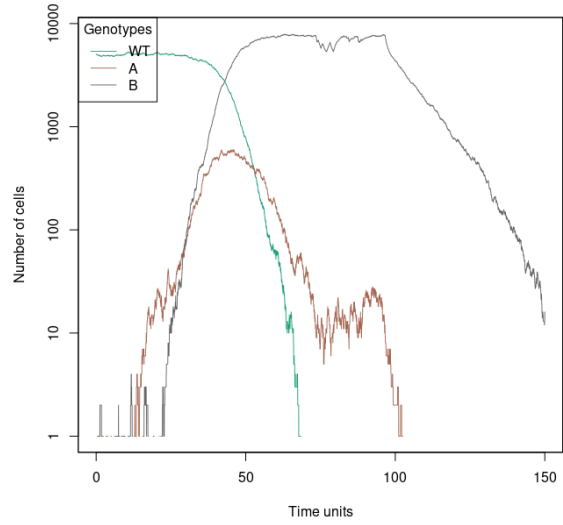
Figura 5.4: Evolución poblacional. Ejemplo 2 variables de usuario
