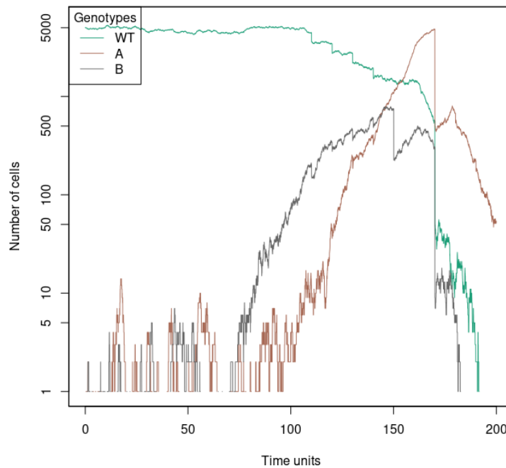
Figura 5.7: Evolución poblacional. Ejemplo 2 terapia adaptativa
