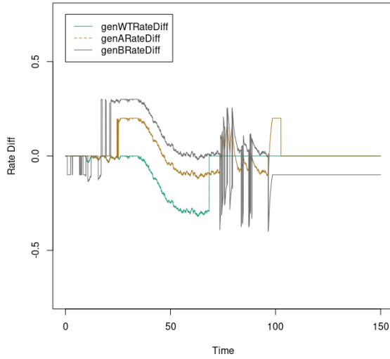
Figura 5.3: Diferencia tasas de nacimiento y muerte. Ejemplo 2 variables de usuario
