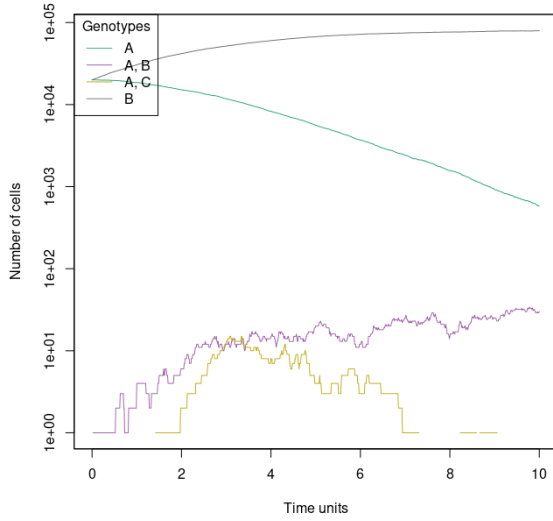
Figura 5.1: Evolución poblacional. Ejemplo 1 variables de usuario
