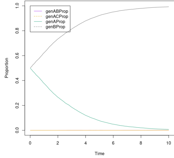
Figura 5.2: Proporción de genotipos en la población. Ejemplo 1 variables de usuario
