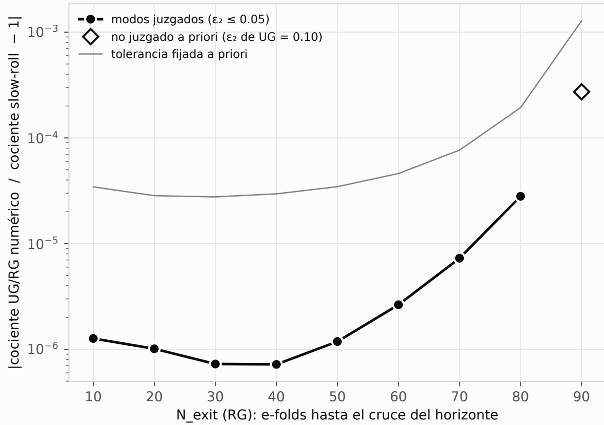
B. UG/RG numérico vs. slow-roll con el fondo de UG
