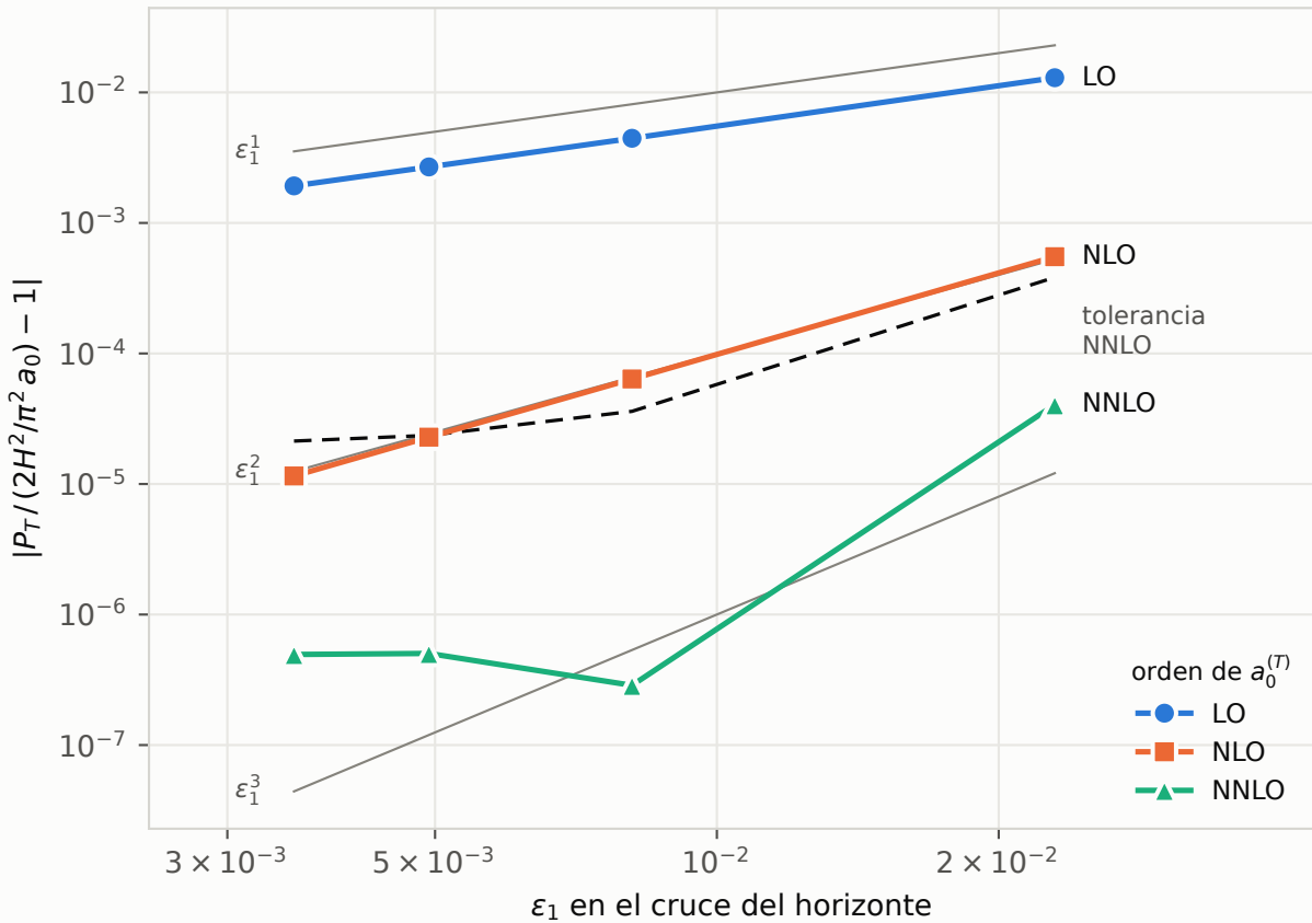
A. RG con \phi^2 : cada orden slow-roll reduce el residuo
