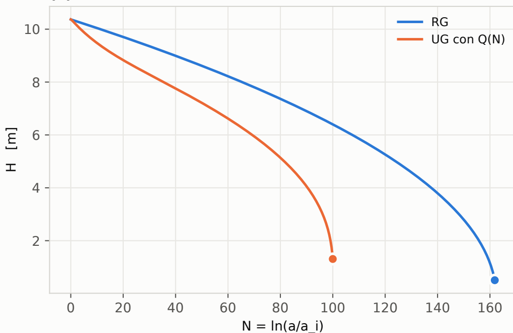
(c) Campo inflatón
