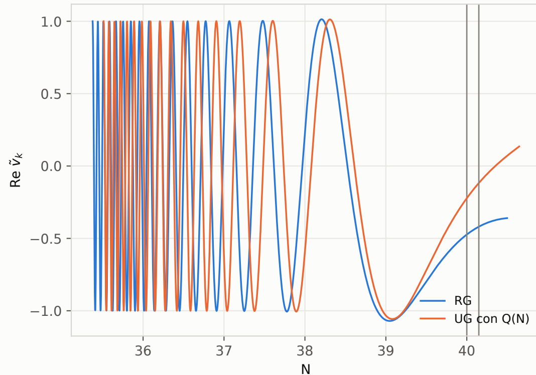
(b) Antes del cruce: oscilaci n de Bunch-Davies
