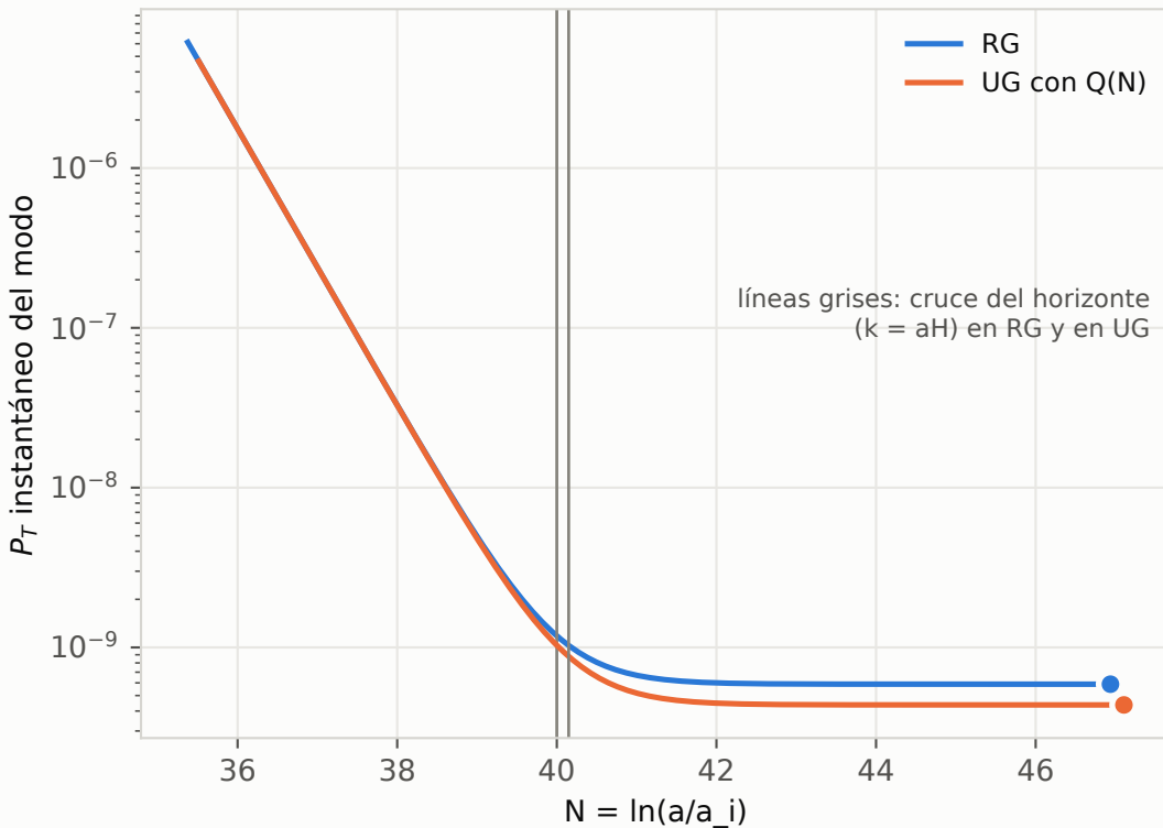
(a) Se congela al salir del horizonte
