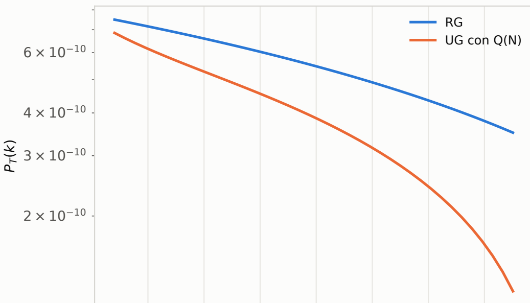
(a) Cuadrático
